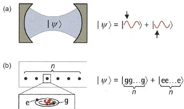
Figur 6. (a) Serge Haroches Schrödinger-killing: Lyset i en kavititet svinger som en helt almindelig sinusbølge, dog i en kvantetilstand, så der bestemte steder i bølgen (f.eks. markeret med pilene) er både en bølgetop og en bølgedal på samme tid. Notationen til højre er fysikerens måde at udtrykke denne såkaldte superposition. (b) David Winelands Schrödinger-killing: Et antal af n ioner er placeret i en ionfælde og kan hver især have sin elektron i en af to elektronbaner, g eller e . I forsøget laves en tilstand, hvor alle ioners elektron er i den samme tilstand, men de er alle i banen g og samtidigt i banen e .
