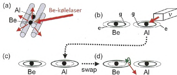
Figur 4. Skitse af David Winelands atomur. (a) En Al- og Be-ion er fanget mellem elektroder i en ionfælde, og Be-ionsens bevægelse nedkøles med en laser. Pga. ionernes elektriske frastødning fjernes bevægelsesenergien (varmen) fra begge ioner, og også Al-ionen kommer til at ligge stille. Vi ønsker at kontrollere, om laserlys med frekvensen \nu opfylder \nu = \nu_0 , og dette lys sendes nu ind på Al-ionen (b), som får sin elektron eksiteret til banen e som vist i (c). Hvis laserlyset er svagt vil denne proces være meget langtvarende og chancen for, at Al-ionen skifter elektronbane, bliver ultra-følsom over for frekvensbetingelsen \nu = \nu_0 . Med særlige laserteknikker, udføres nu en swap operation, dvs. Be-ionen bliver eksiteret, betinget af at Al-ionen var eksiteret. Den eksiterede Be-ion i (d) kan effektivt udføre kvantespring og udsende lys, som kan detekteres.
