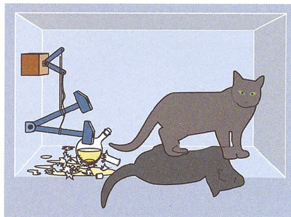
Figur 5. I en lukket kasse er en Geigertæller placeret nær en så lille mængde radioaktivt materiale, at sandsynligheden for et udslag i løbet af en time er 50 %. Hvis et radioaktivt henfald registreres, udløses en hammer, der smadrer en flaske med blåsyre, der vil dræbe en kat, som således har en fifty-fifty chance for at overleve efter en time. Schrödinger fandt det absurd, at en bølgeteori skulle kunne redegøre for, hvad der foregår i kassen, for i sådan en teori ville katten efter en time (inden kassen åbnes), være beskrevet som både levende og død, og dens skæbne ville først afgøres tilfældigt, idet kassen åbnes. Paradokset stiller spørgsmålet: Hvor går grænsen mellem bølgefunktionens "både-og" og måleresultaternes "enten-eller"?
