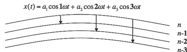
Figur 2. En klassisk baneurve opløst i Fourierkomponenter [2]. Ifølge korrespondensprincippet svarer enhver tilladt overgang mellem stationære baner til en af den klassiske bevægelses harmoniske komponenter.
