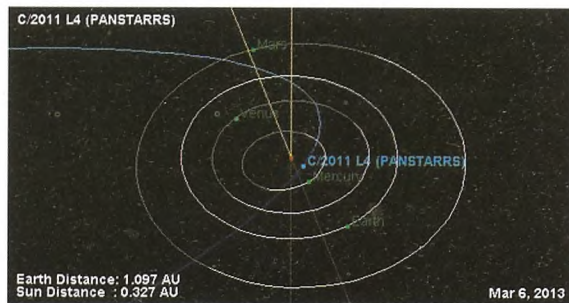
Figur 3. Kometens bane gemmen den inderste del af Solsystemet.
